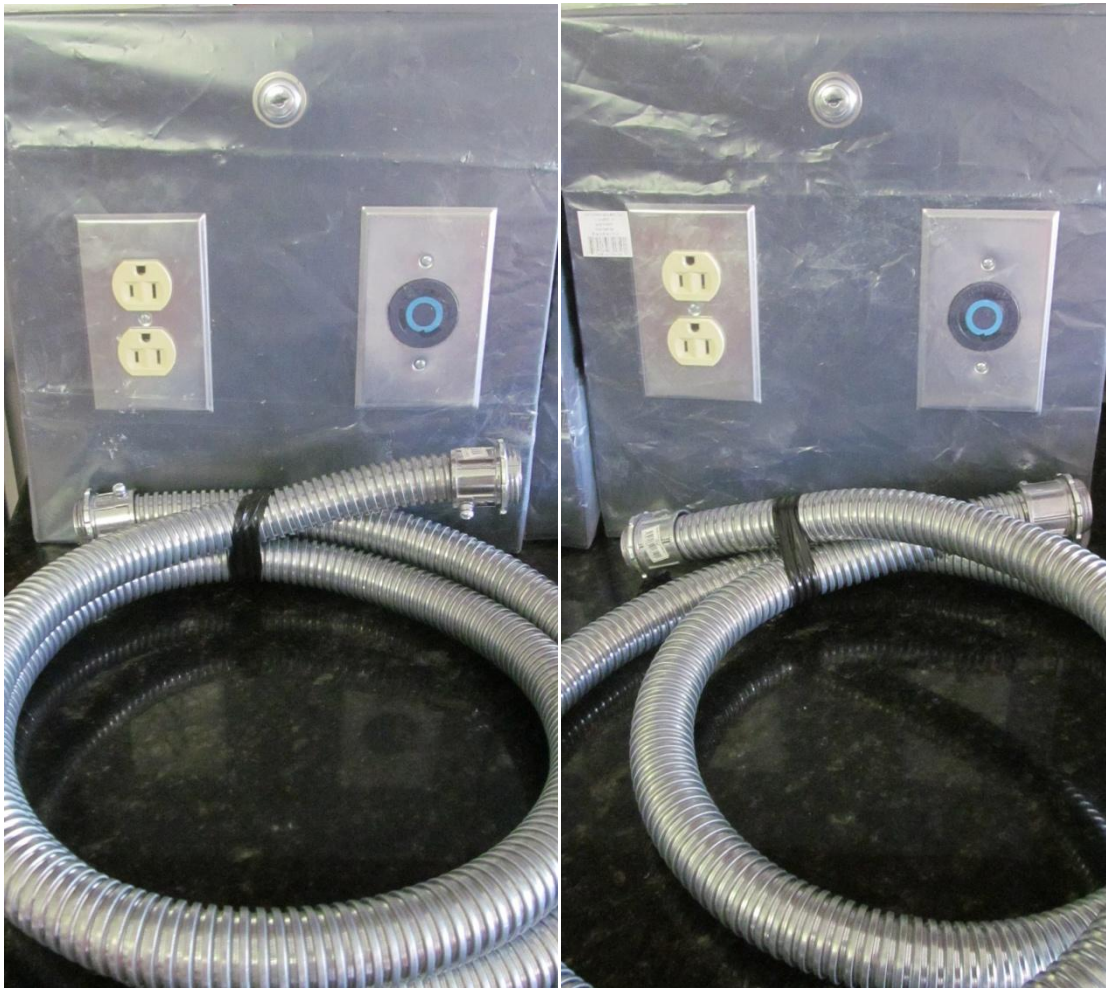
Anexo 6: Embalaje y flexible 1" con conectores 1" para instalación.
